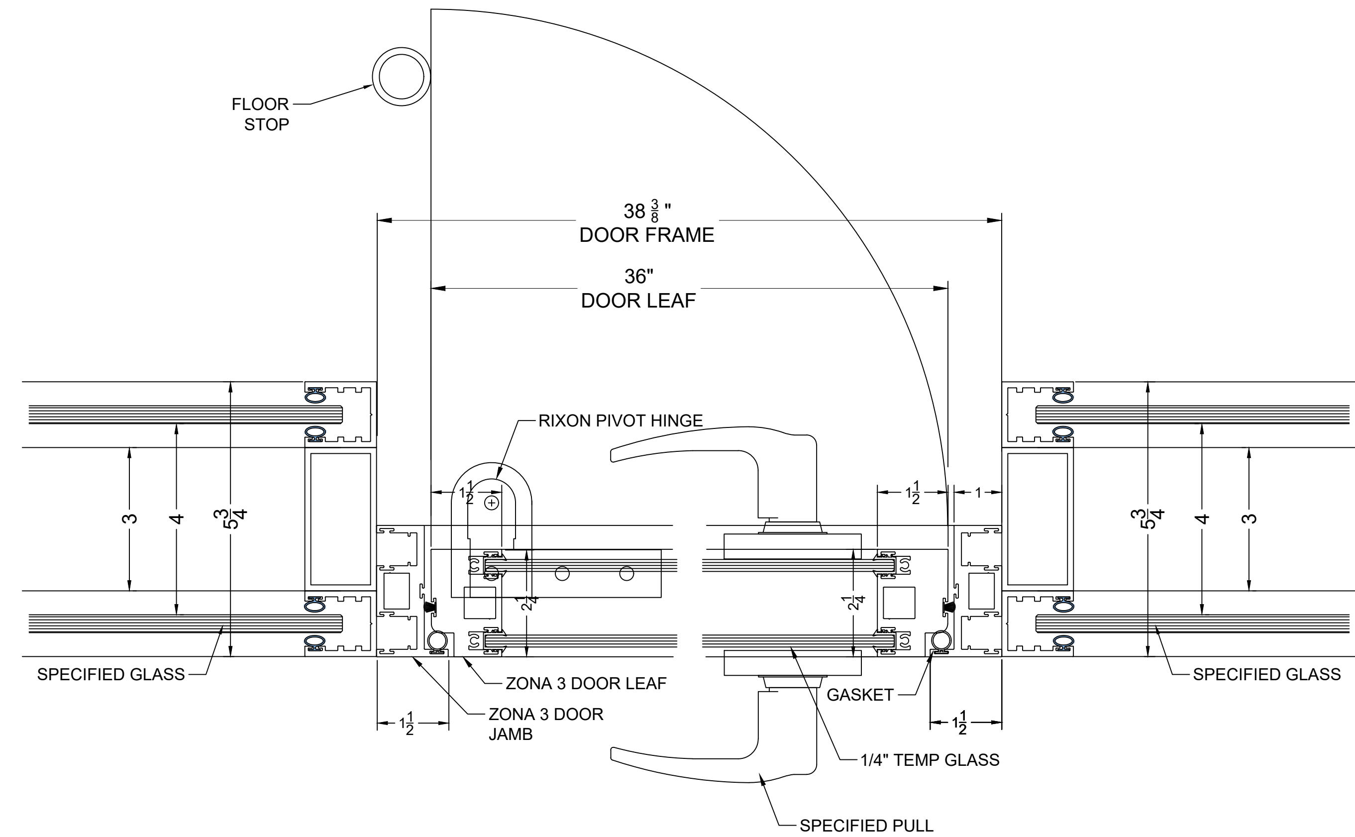
6 DOOR BTW FIXED GLASS SIDE LITES HORZ. SECT. @DBL GLZD DOOR W/LOCKSET 51 STC
