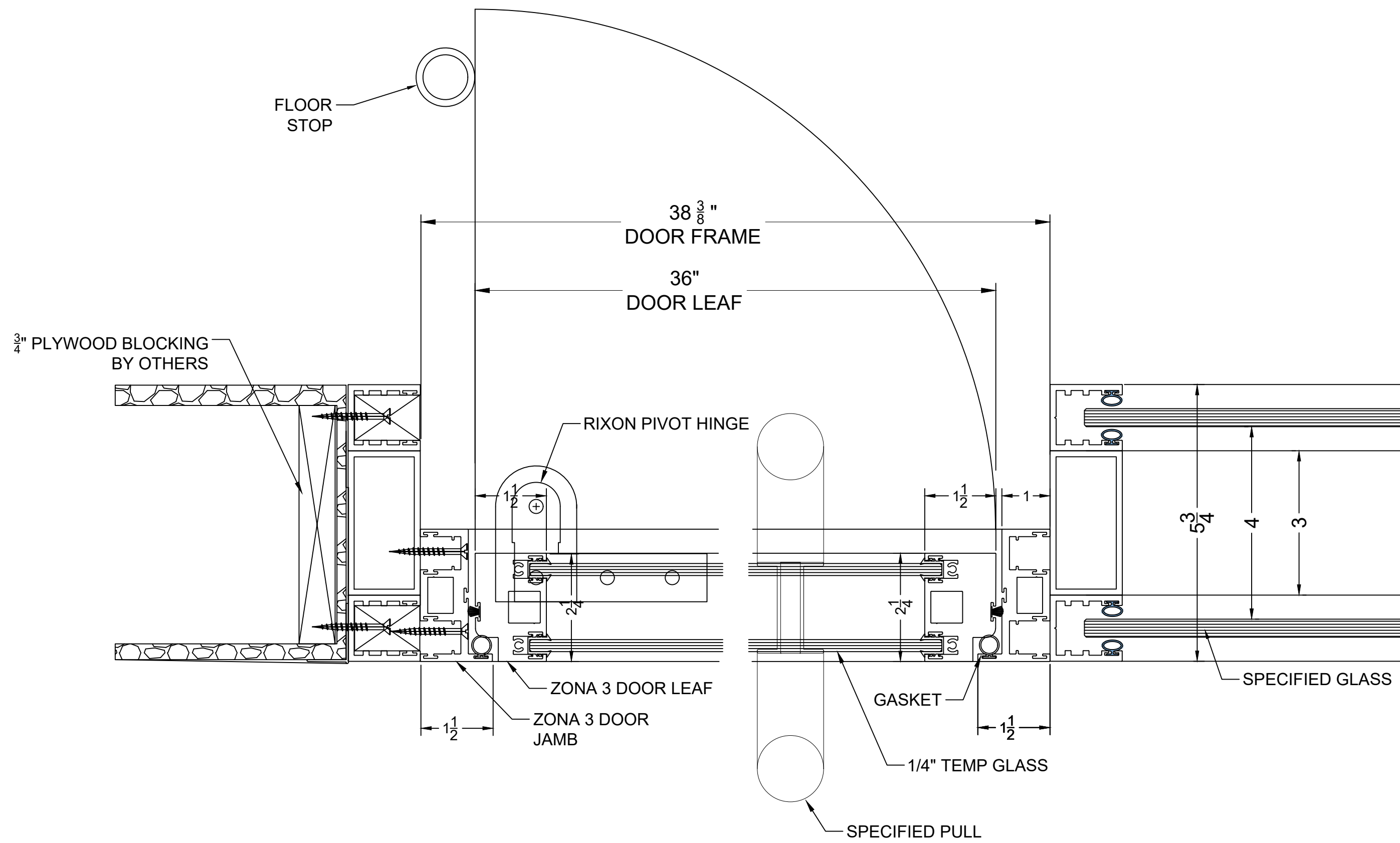
5 DOOR @ NIB WALL HORZ. SECT. @ DBL GLZD DOOR W/PULL 51 STC
