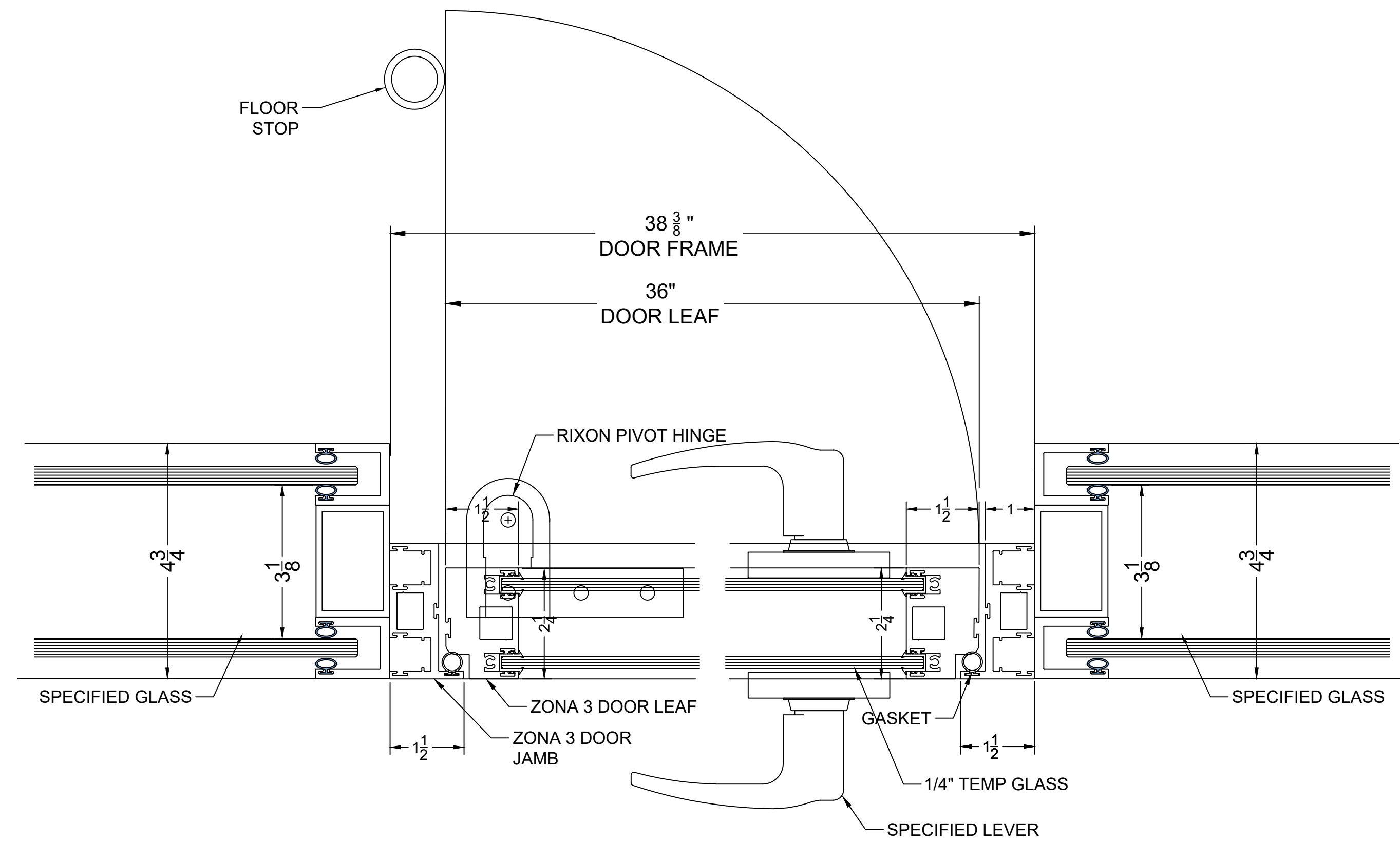
6 DOOR BTW FIXED GLASS SIDE LITES HORZ. SECT. @DBL GLZD DOOR W/LOCKSET 49 STC
