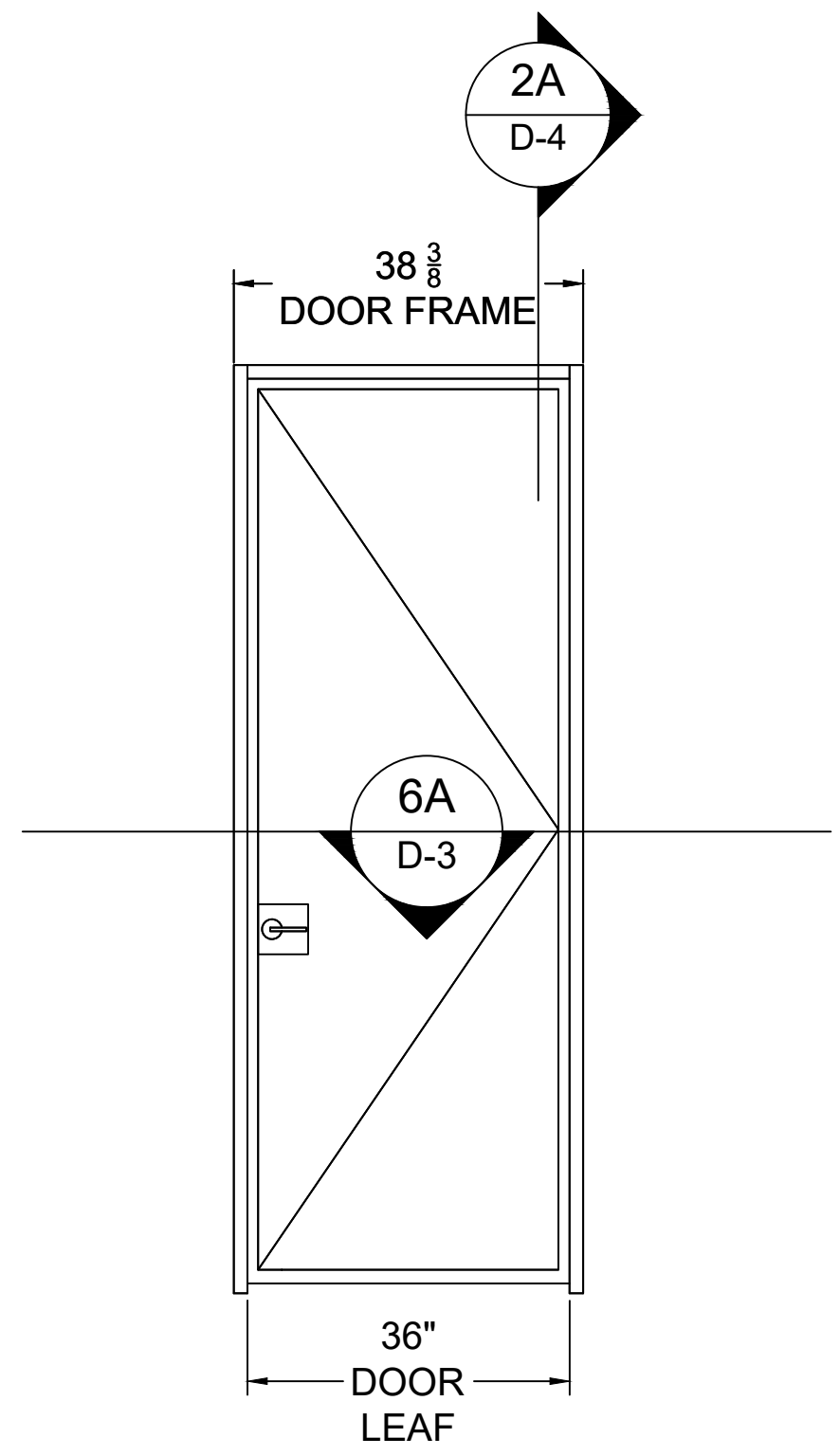
47 WOOD DOOR W LOCKSET
