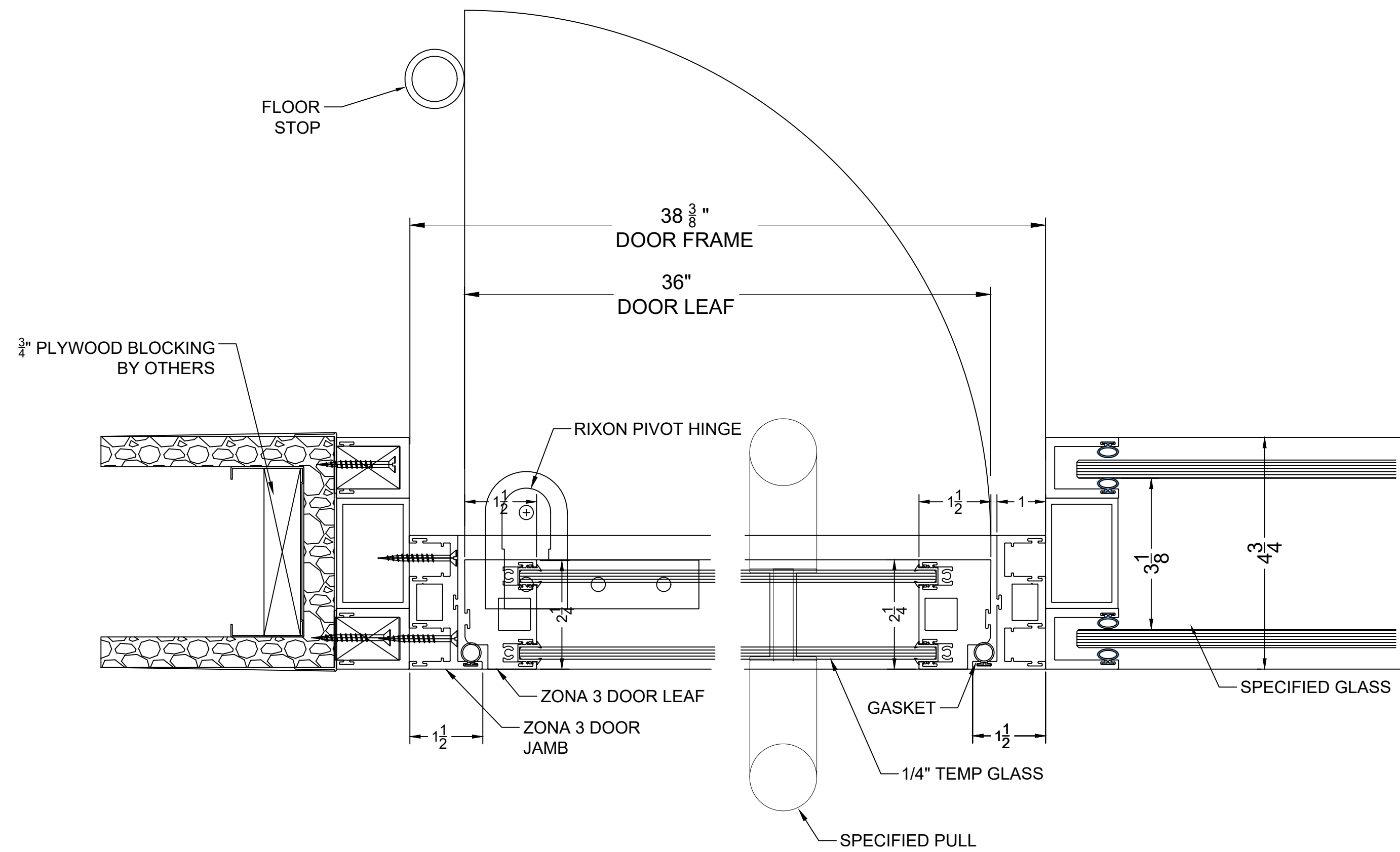
5 DOOR @ NIB WALL HORZ. SECT. @ DBL GLZD DOOR W/PULL 49 STC
