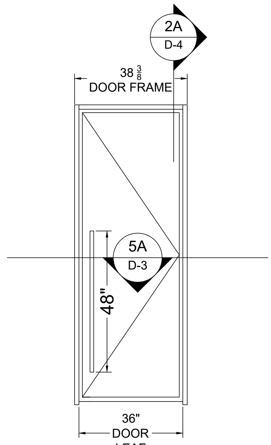
47 WOOD DOOR W PULL EXAMPLE
