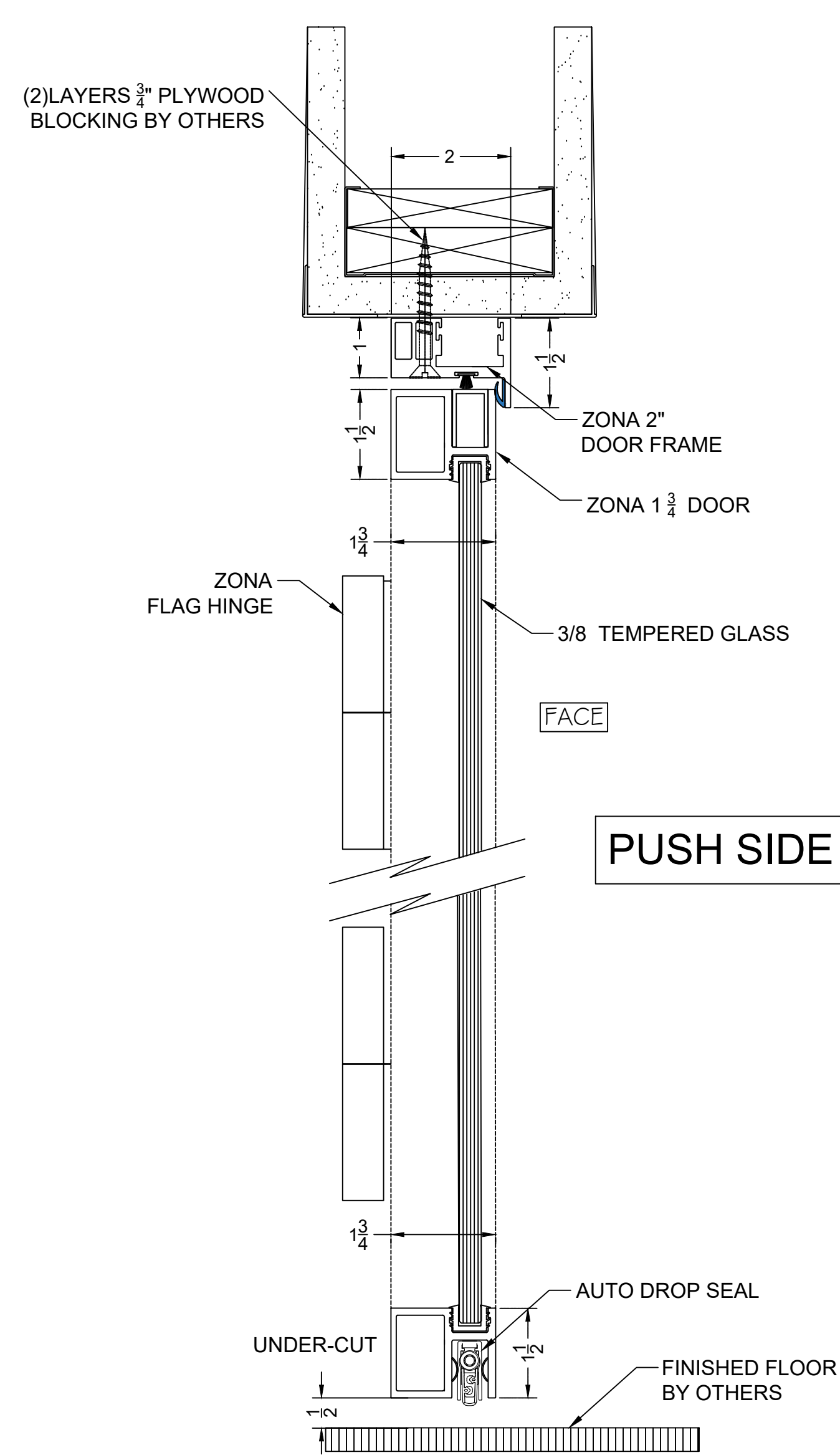
2 ZONA FLAG HINGE - FREE-SWING DOOR VERT. SECT. @ DOOR
