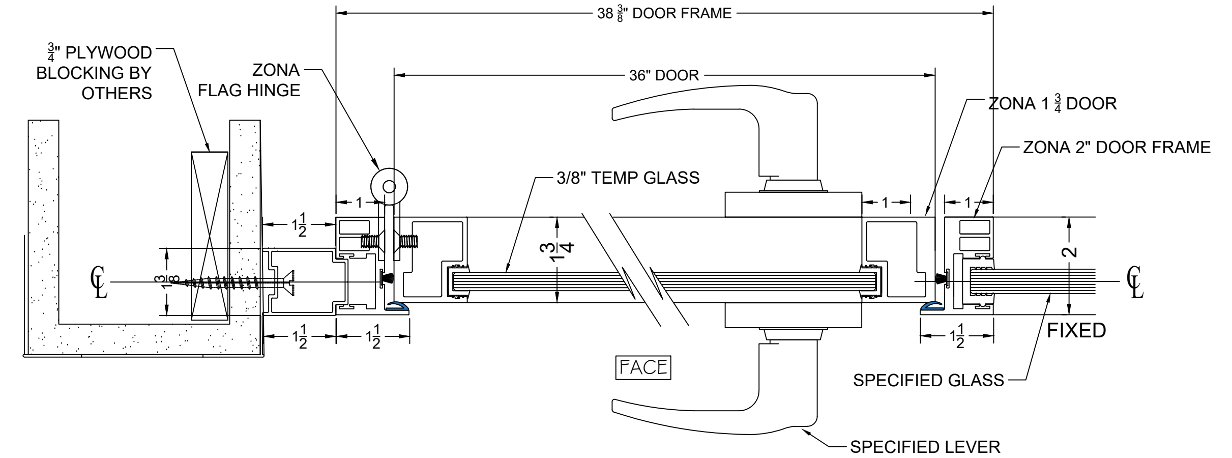
5 DOOR @ DIVIDER WALL HORZ. SECT. @ DOOR W/LOCKSET
