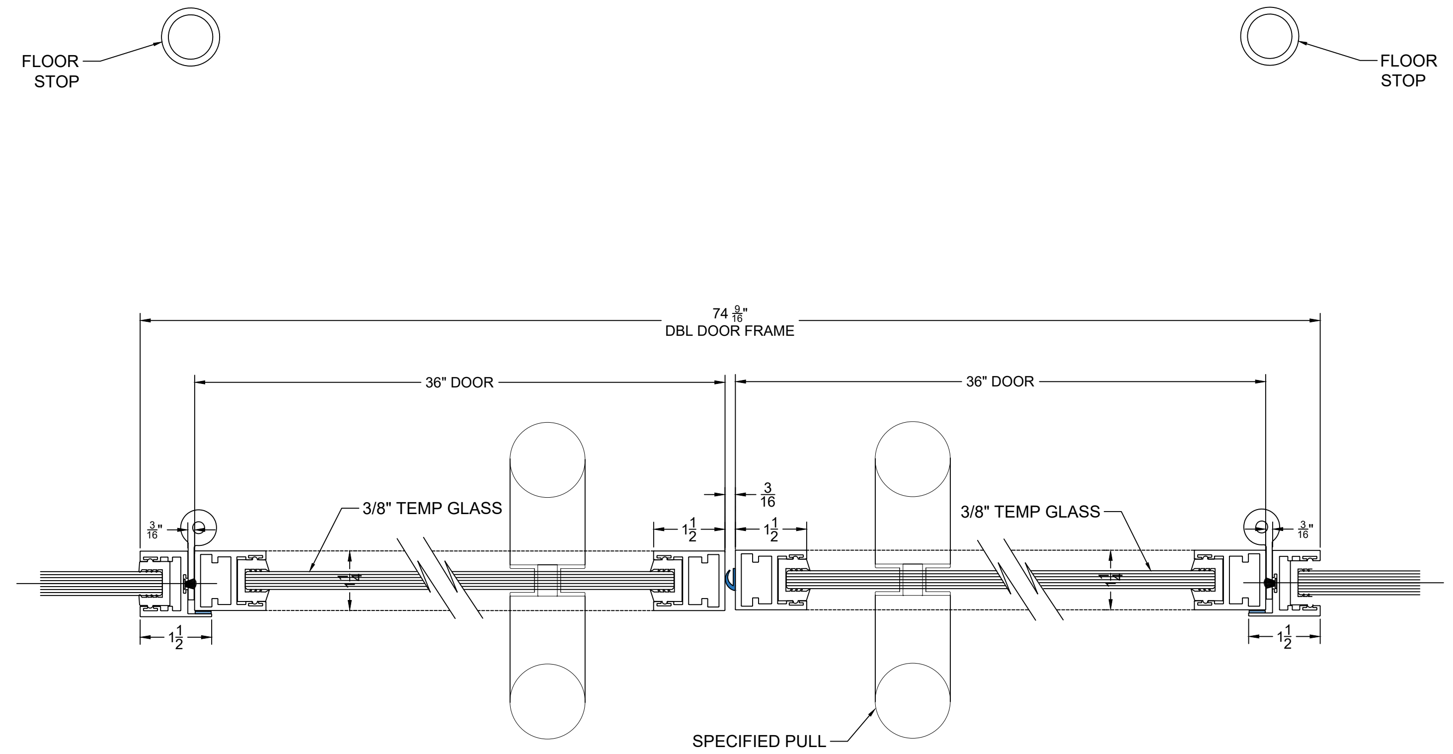
5 HORZ. SECT. @ DOUBLE DOOR DOUBLE DOORS W/GLASS SIDE LITES
