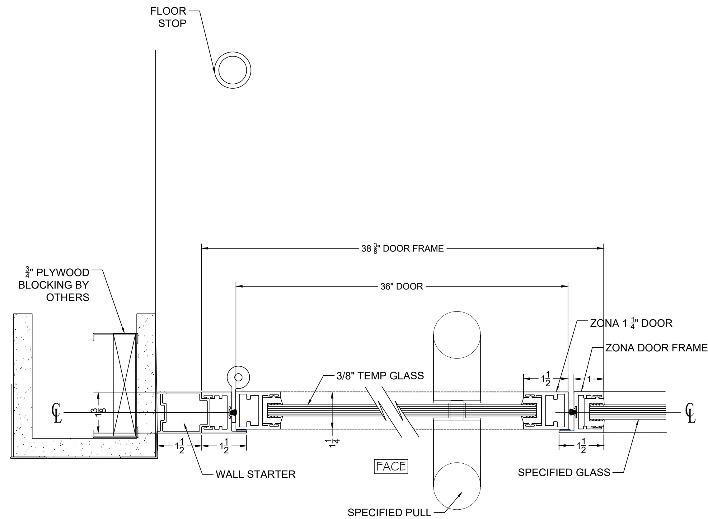
4 HORZ. SECT. @ DOOR DOOR TO DIVIDER WALL
