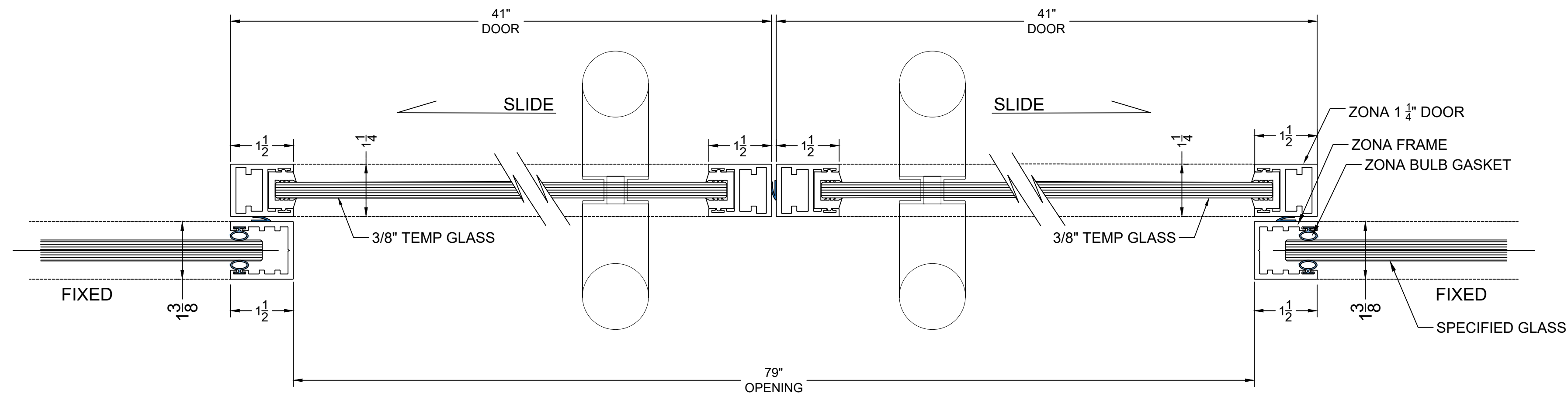
9 DOOR BTW FIXED SIDE LITES HORZ. SECT @ SINGLE SLIDING DOOR
